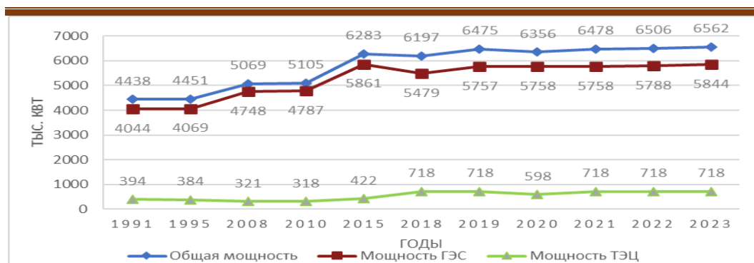
Рисунок 1. Изменения мощностей генерации. Синяя (верхняя кривая) - общая мощность, красная (вторая кривая) - мощность ГЭС, зелёная (нижняя кривая) - мощность ТЭЦ.
